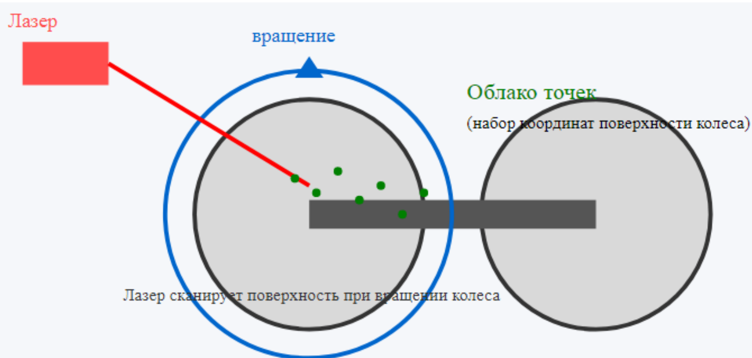
Рисунок 3 – Лазерное 3D-сканирование вращающейся колесной пары и формирование облака точек
